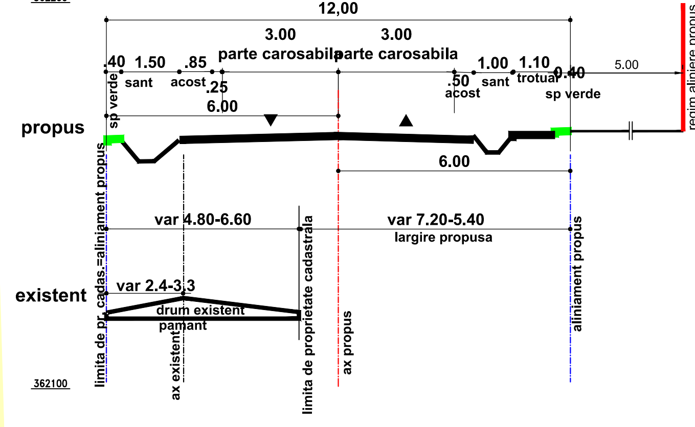
PROFIL TRANSVERSAL TIP -d-d la De 435/34
