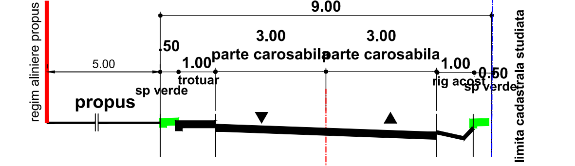
PROFIL TRANSVERSAL TIP -e-e la drum nou propus
